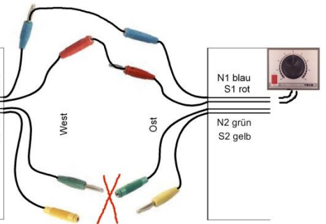
Ansicht von der Modulunterseite
