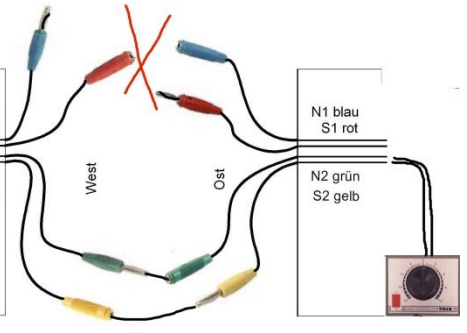
Ansicht von der Modulunterseite
